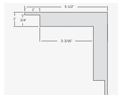
Kleer Konceal® Corner #5559
