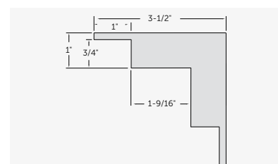
Kleer Konceal® Corner #5552
