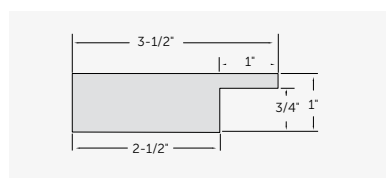
Kleer Konceal® Trimboard #5553
