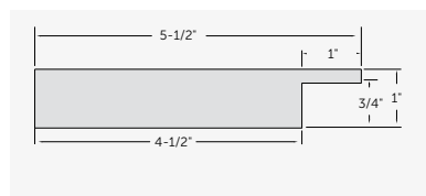
Kleer Konceal® Trimboard #5561
